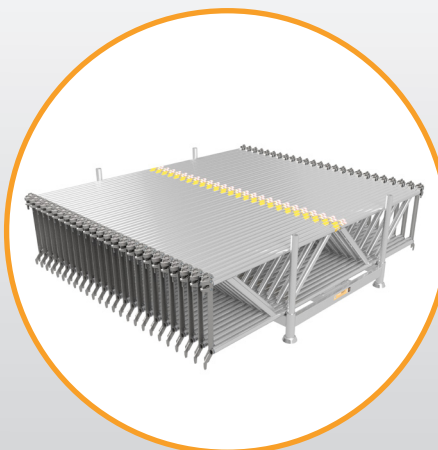
MonZon Guardrails™ -suojakaiteiden paino on 414 kg, mukaan lukien 225 cm:n lava.
