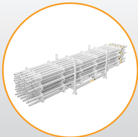
Pystytolpat , joiden paino 320 kg, mukaan lukien lava 80. Kuorma-auton täyteen kuormaan mahtuu 1 716 kappaletta, joiden kokonaispaino 10 574 kg verrattuna 27 334 kg:n painoon (300 cm:n pystytolpat, jotka valmistettu teräksestä), mukaan lukien 80 ja 65 cm:n lavat.
