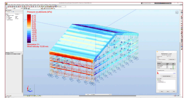
Autodesk Robotin tuulitunnelien simulointi ja vahvuuslaskelmat antavat helposti kaikki tuulikuormat EN-1991-4: n mukaisesti.
