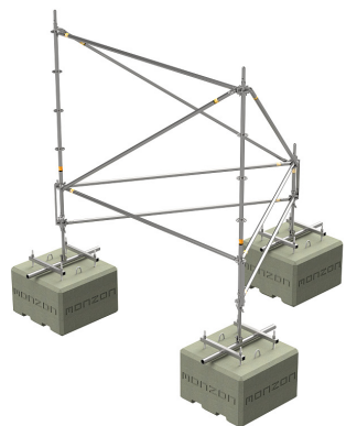
PROJEKTIN KYLTTI BILLBOARD™ (3 × 4 m)
