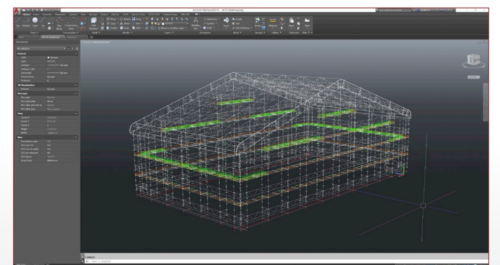
Analysoi tulos SCAFFCAD™ -järjestelmällä standardin SS-EN 16508: 2015 eurooppalaisten vaatimusten mukaisesti.
