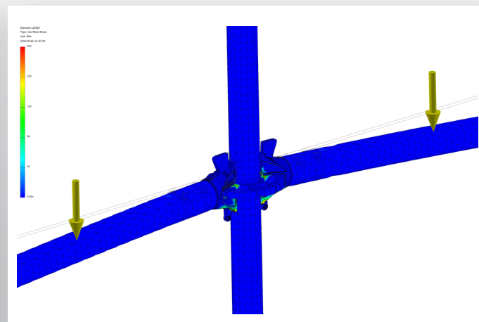
O-juoksun/pystytolpan liitännän momentin (My+) FEA.
