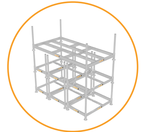
Alumiinilavoja on kolmea eri kokoa, ja ne voidaan pinota..
