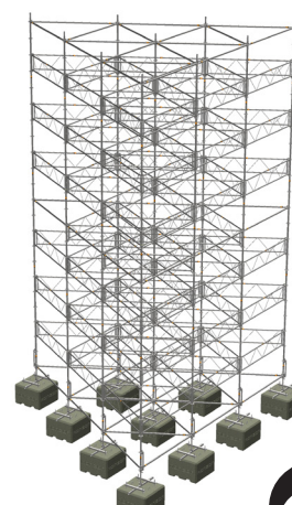
PROJEKTIN KYLTTI BILLBOARD™ (8 × 11 m)
