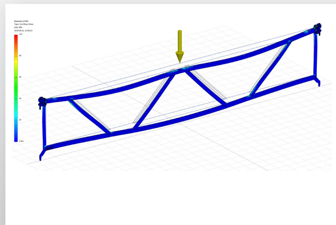
MonZon Guardrail™ -suojakaiteen FEA (kuorma tasaisesti jakautunut).
