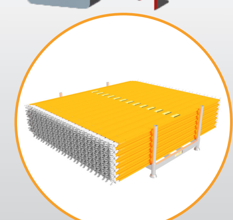
MonZon Toeboards™ -jalkalistojen paino on 1 104 kg, sisältäen 225 cm:n lavan.
